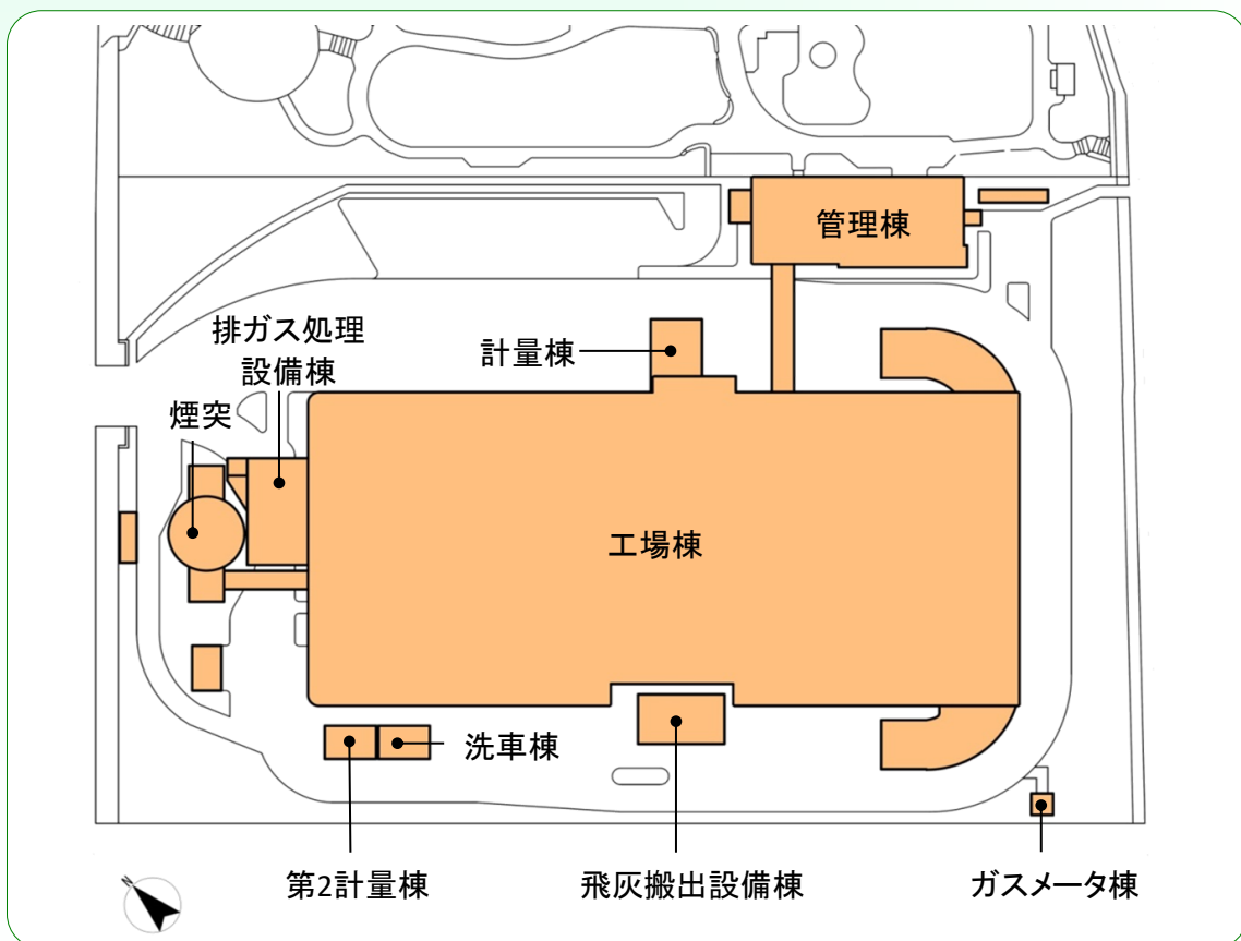
解体施設(既存清掃工場)配置図
