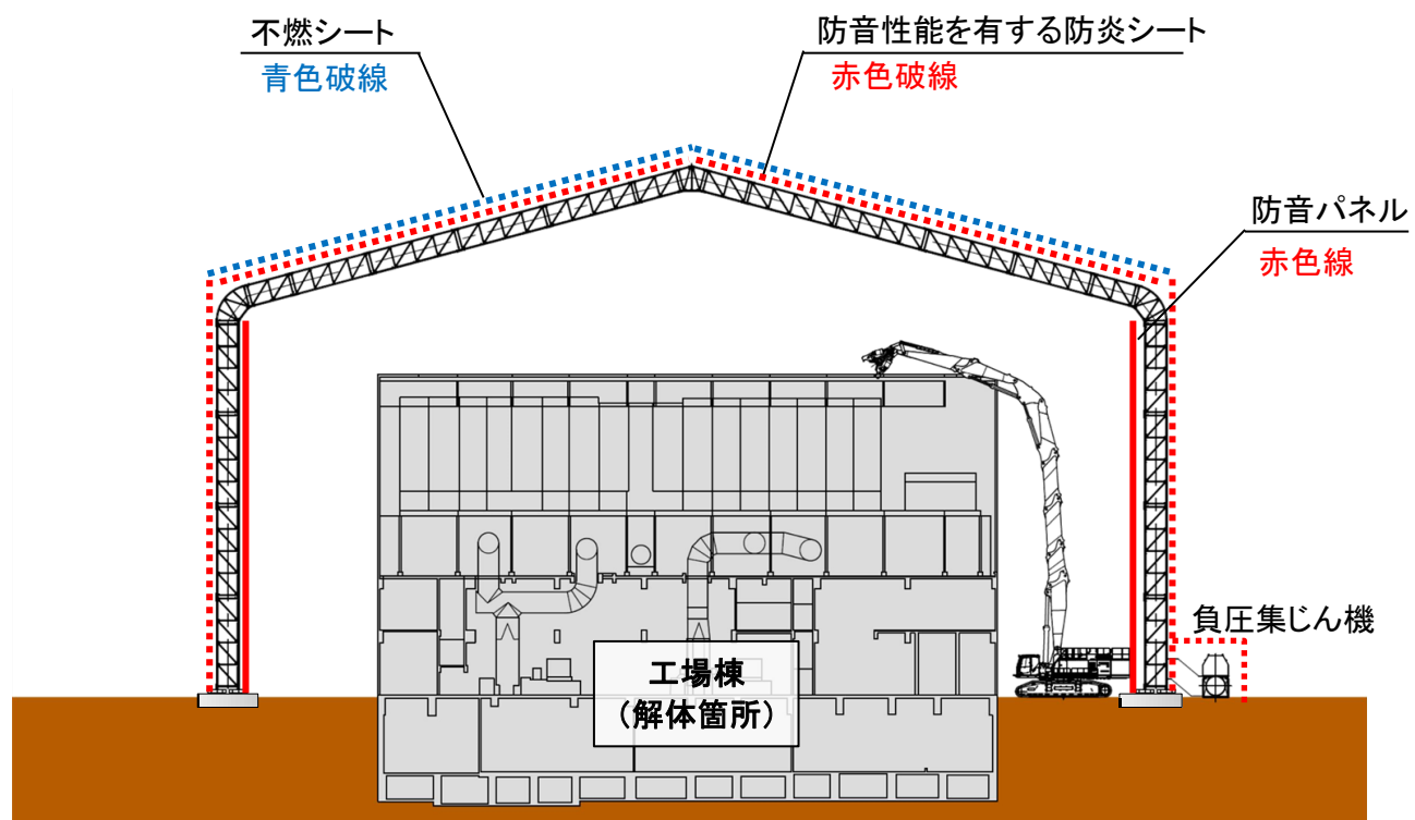
工場棟解体作業のイメージ図
