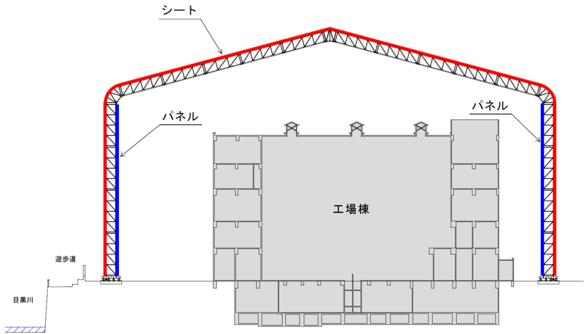
断面図
