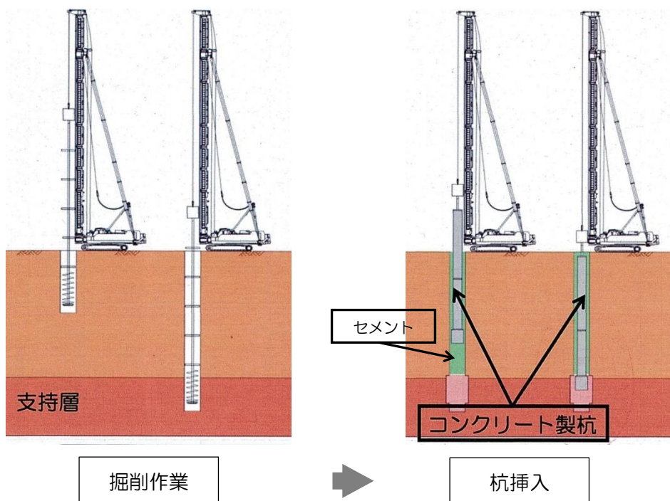
作業手順 断面図 (イメージ図)
