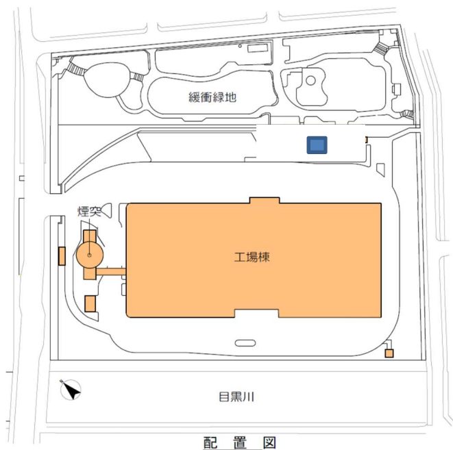
配置図
