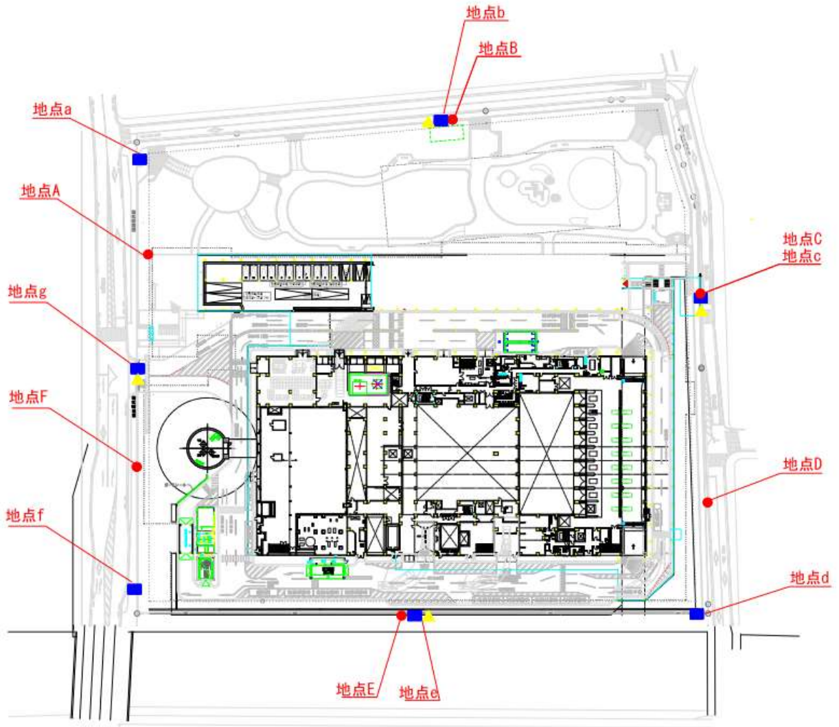
騒音測定点図 (●が調査地点)
